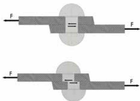
Obr. stříhové napětí
