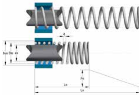
Příklad technických informací pro výpočet tlačných pružin
