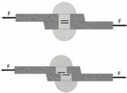
Fig. schuifspanning
